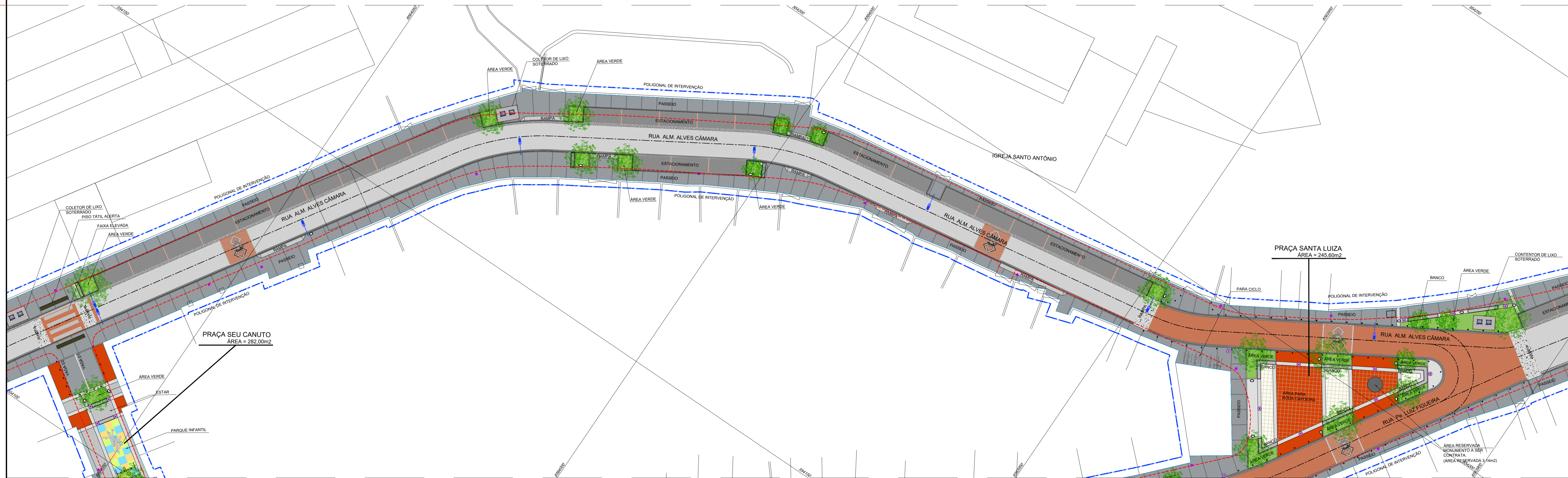
PROJETO BÁSICO URBANÍSTICO - TRECHO 05 ESC: 1:250
