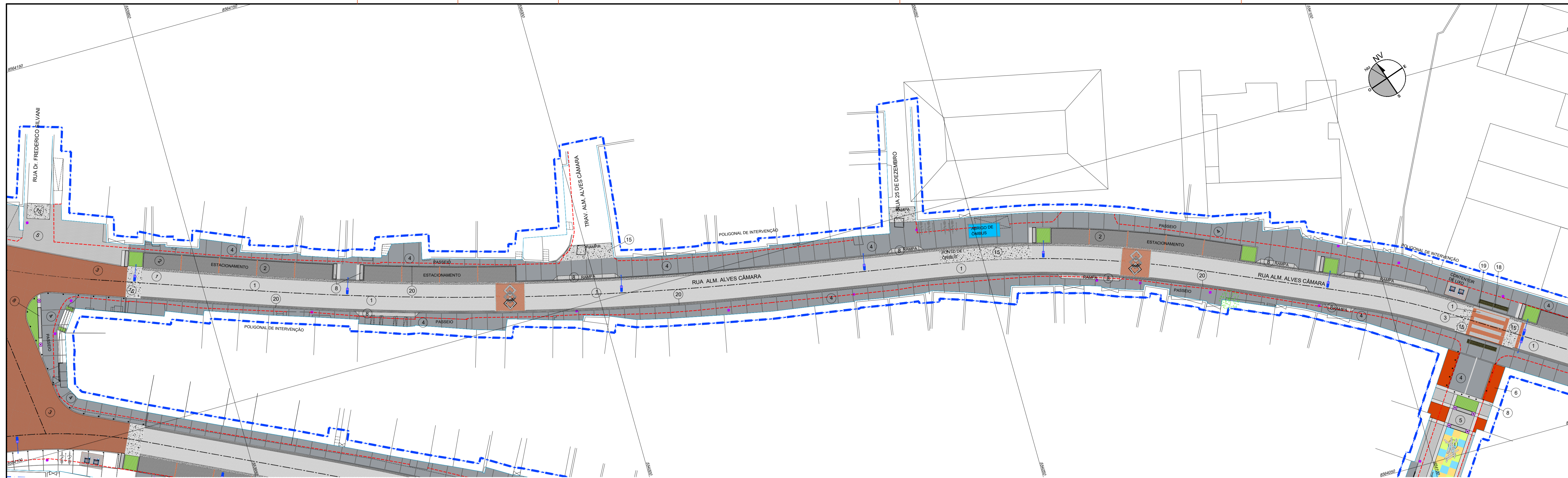
PLANTA GERAL DE PAVIMENTAÇÃO - TRECHO 04 ESC: 1:250
