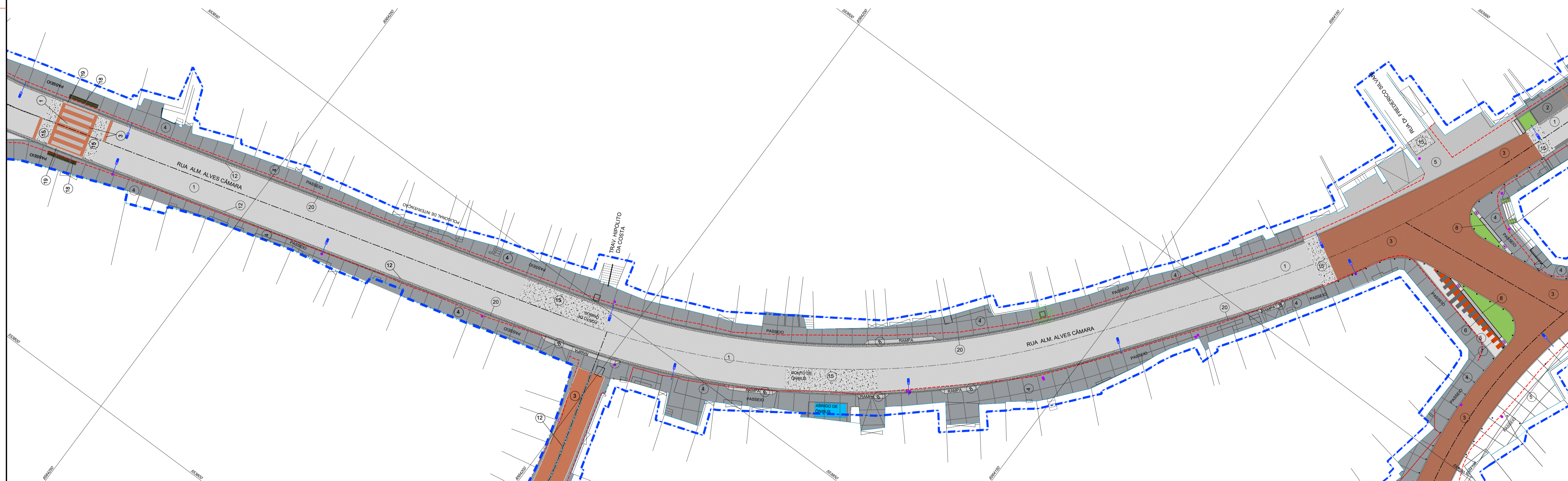
PLANTA GERAL DE PAVIMENTAÇÃO - TRECHO 03 ESC: 1:250
